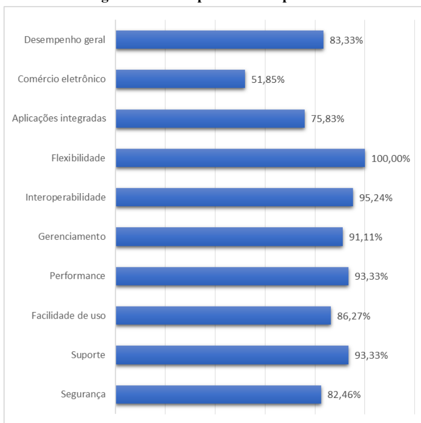
Figura 7 – Desempenho obtido pelo Plone
