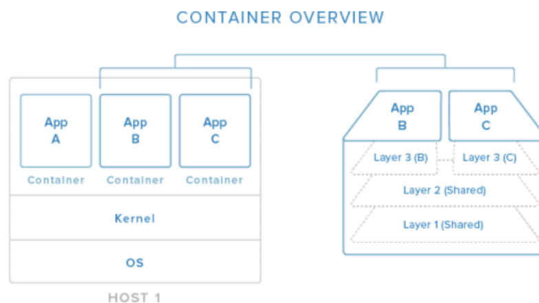
Figura 11 – Esquema explicativo da estrutura de containers
