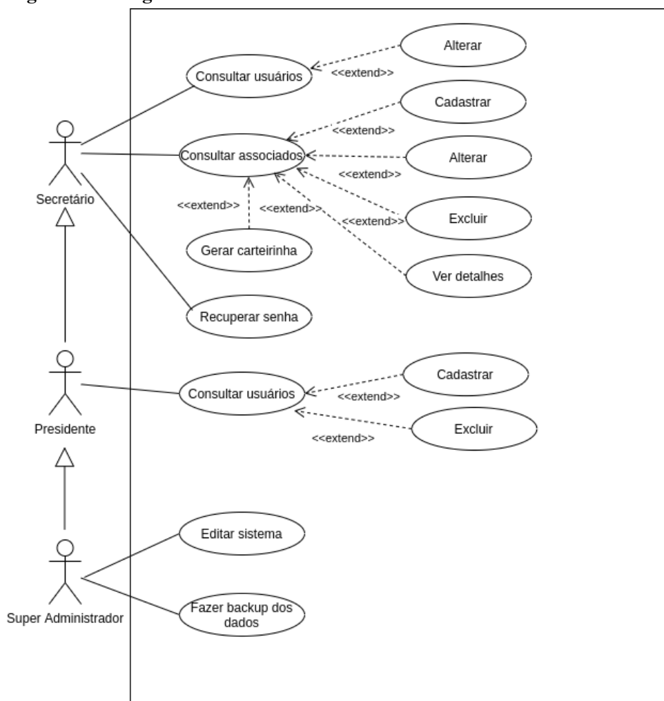
Figura 15 – Diagrama de casos de uso do sistema de associados da Kuruatuba
