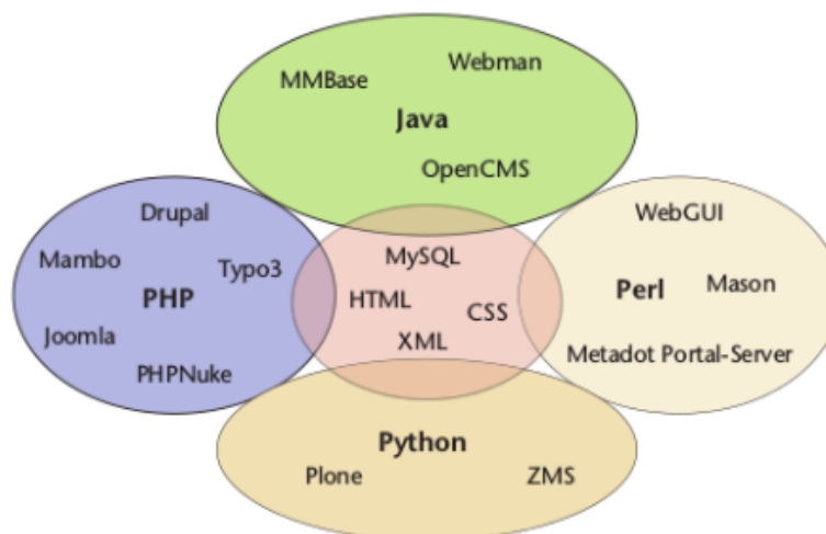
Figura 2 – Sistemas de Gerenciamento de Conteúdo da web de código aberto e tecnologias relacionadas
