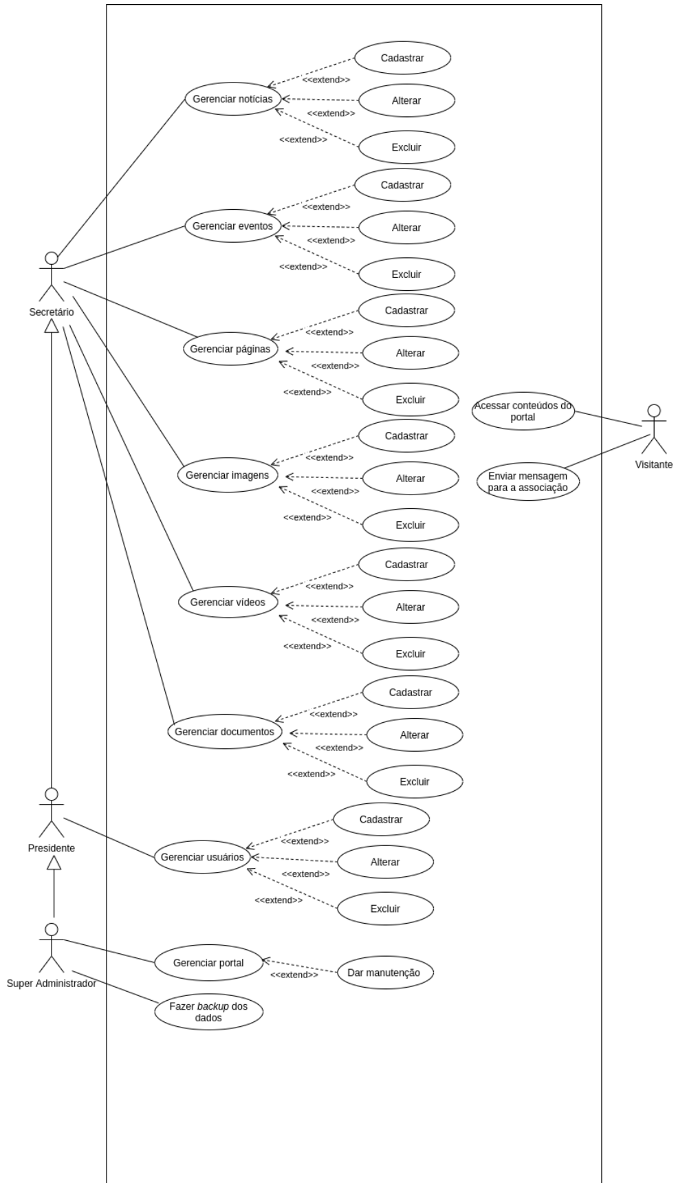
Figura 14 – Diagrama de casos de uso do portal da Kuruatuba
