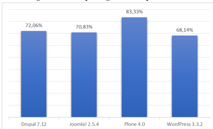
Figura 9 – Desempenho geral obtido pelos sistemas
